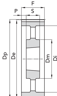
ESEC. 12
