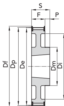
ESEC. 6F
