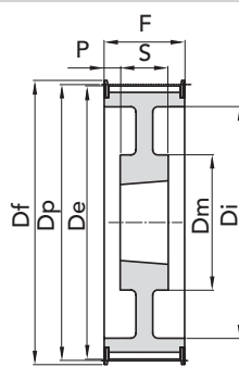
ESEC. 10F
