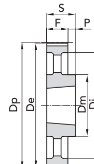
ESEC. 8
