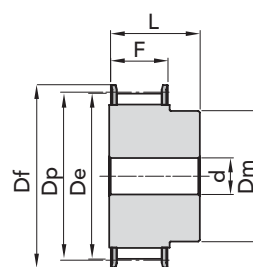
ESEC. 1F
