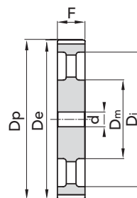
ESEC. 5
