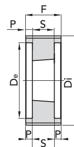
ESEC. 4
