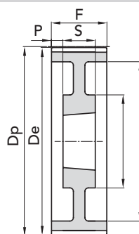
ESEC. 11
