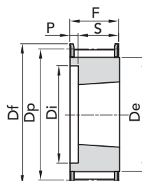
ESEC. 2F
