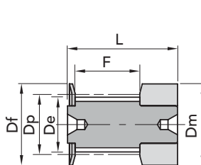
ESEC. 0F
