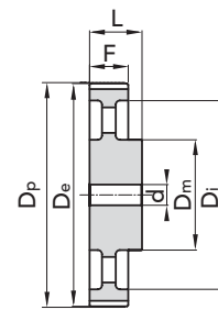
ESEC. 4
