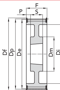
ESEC. 10F
