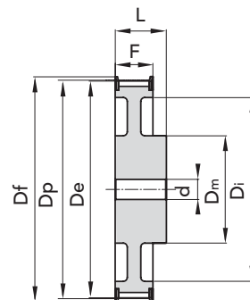
ESECUZIONE 2F
