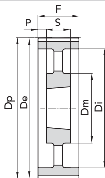
ESEC. 12
