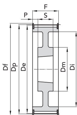
ESEC. 10F
