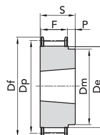
ESEC. 5F
