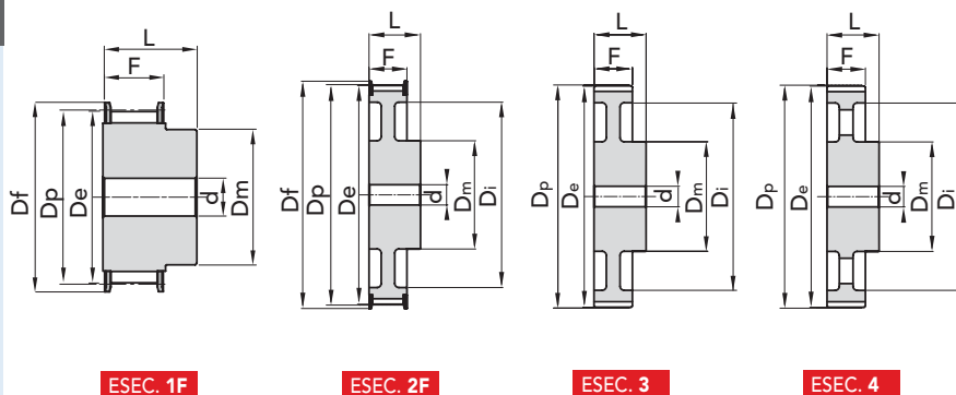
ESEC. 1F
