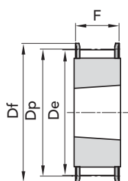
ESEC. 1F
