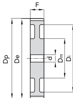
ESECUZIONE 7
