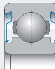
DOUBLE DÉFLECTEUR (suffixe ZZ)
